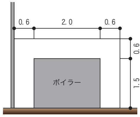
(立面図)
